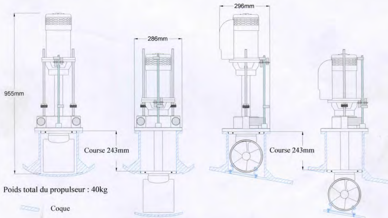
VIP 150 12/24V : dimensions principales
