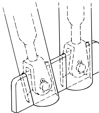
Röstjärnet är bredare än röret. Röret måste slitsas.
