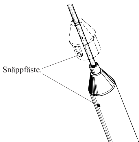
Röstjärnet ryms inne i röret.
