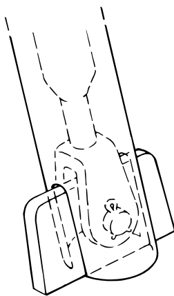
Röstjärnet är bredare än röret. Röret måste slitsas.
