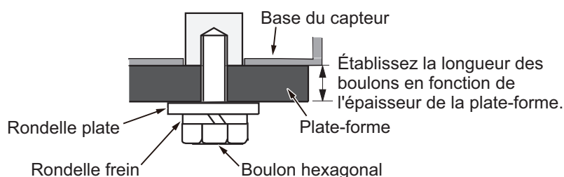
Épaisseur de la plate-forme et boulon à utiliser
